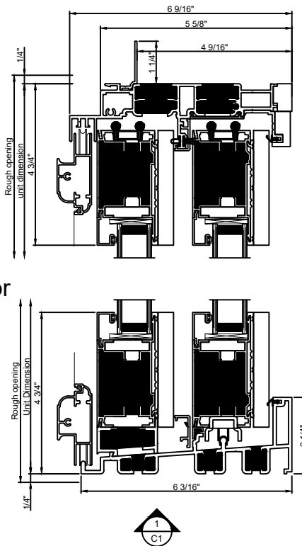
Door cut sections 1 : 4
