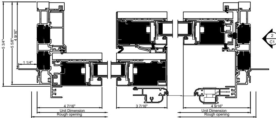
Door cut sections 1 : 4
